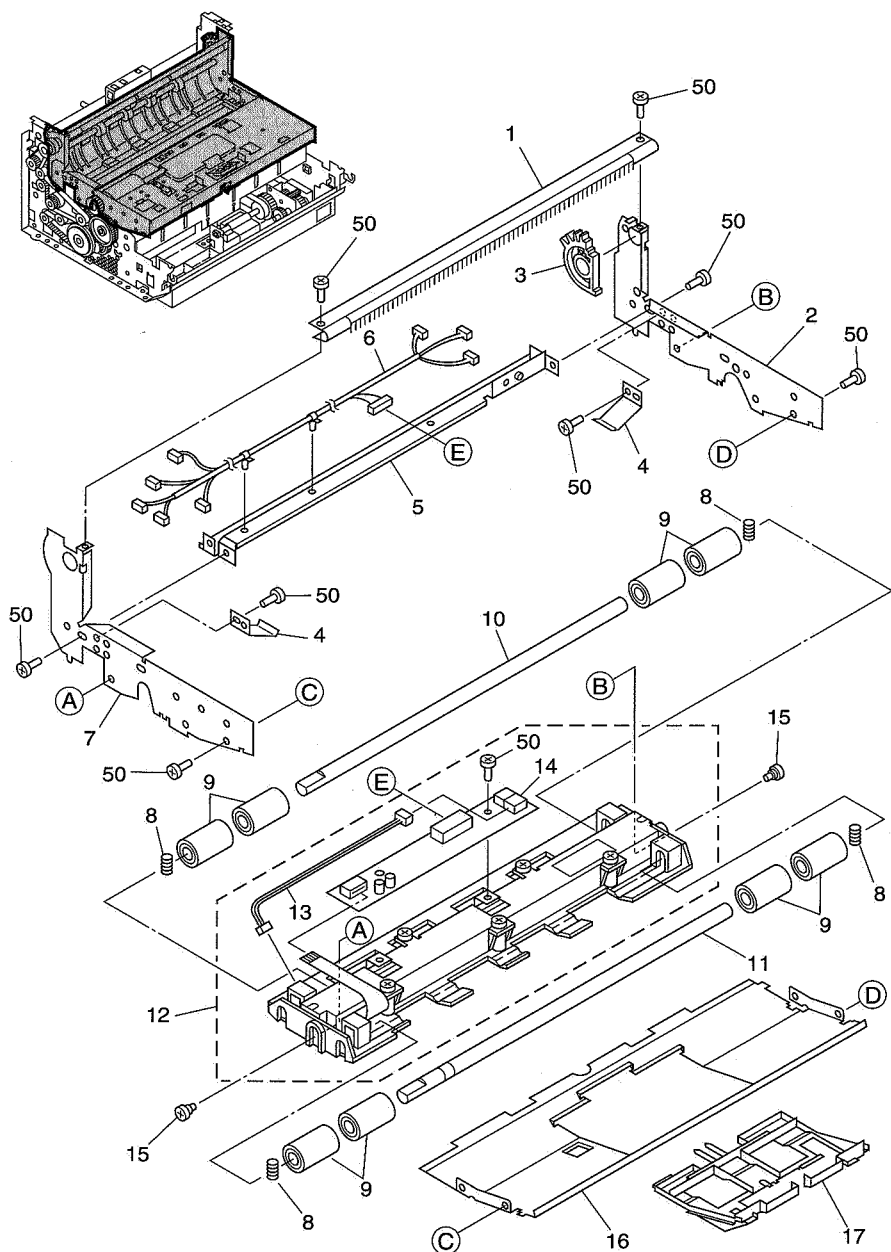
上搬送部-1
