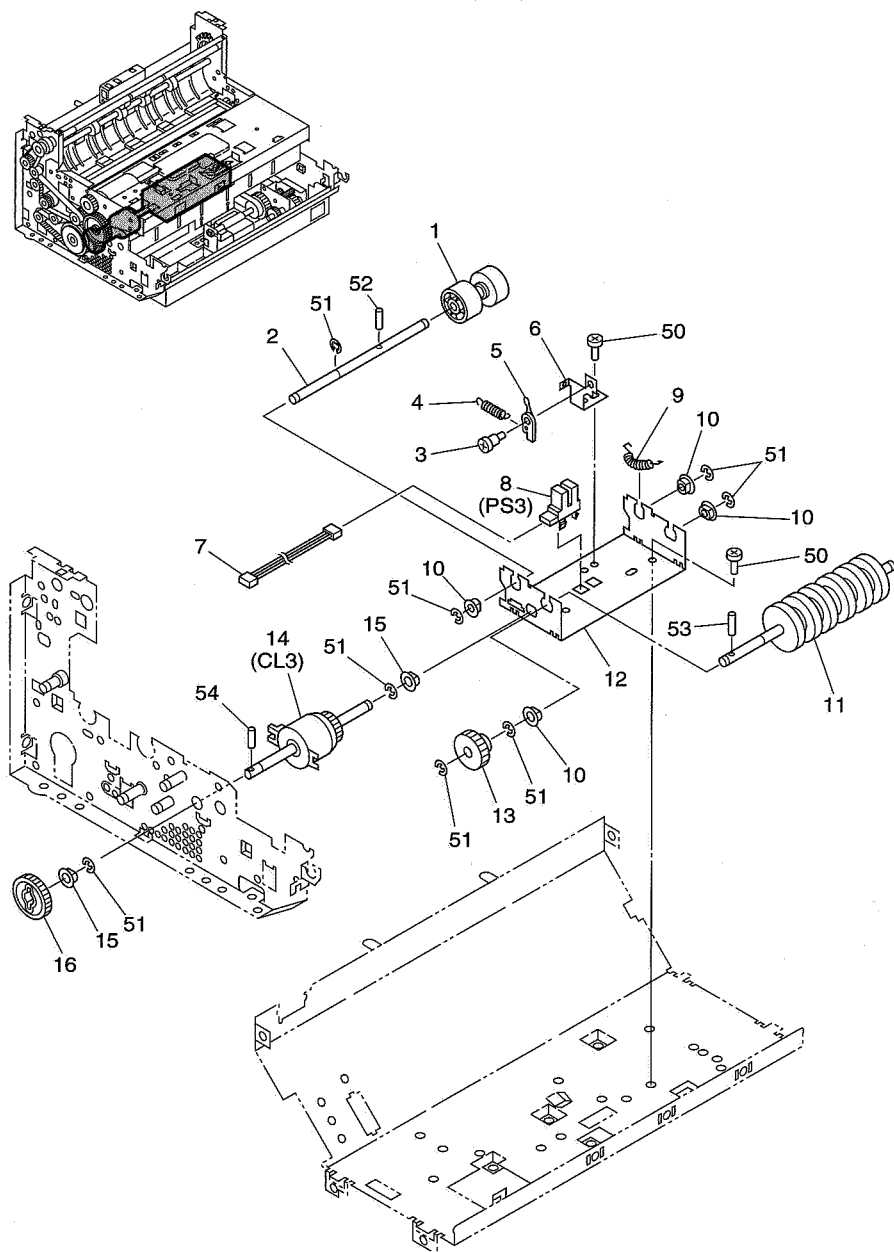
下搬送部-2
